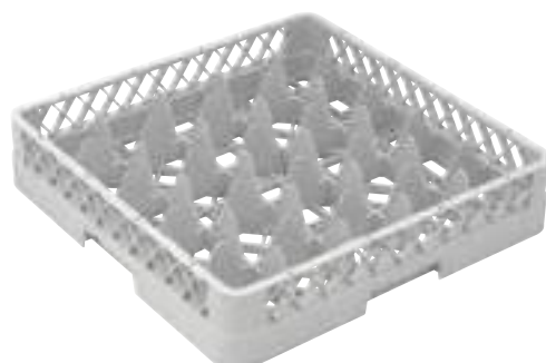
12626 BASE 25 SCOMPARTI GRIGIA cm 50x50 Dimensione scomparti cm 8,8x8,8 H 8,8
